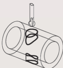
偏心交差穴
